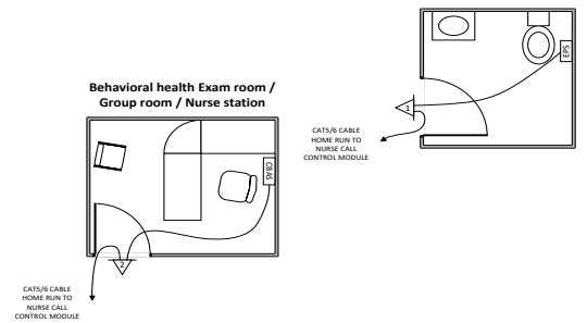
Patient Toilet
