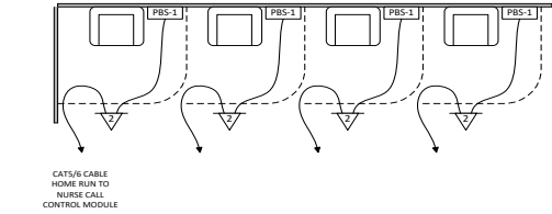
Patient Toilet
